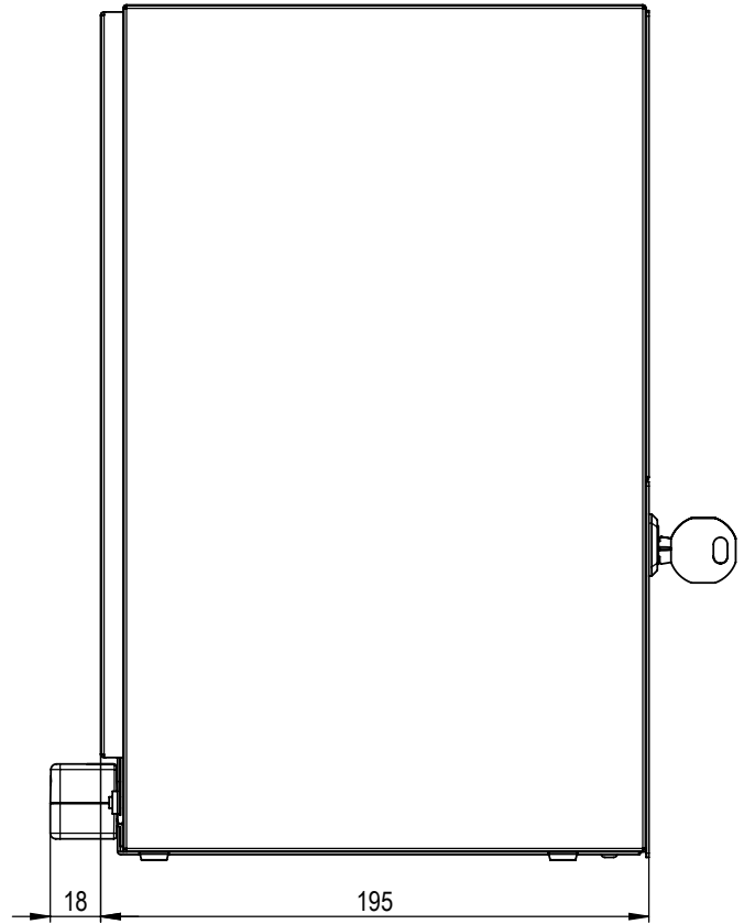
Seitenriss
