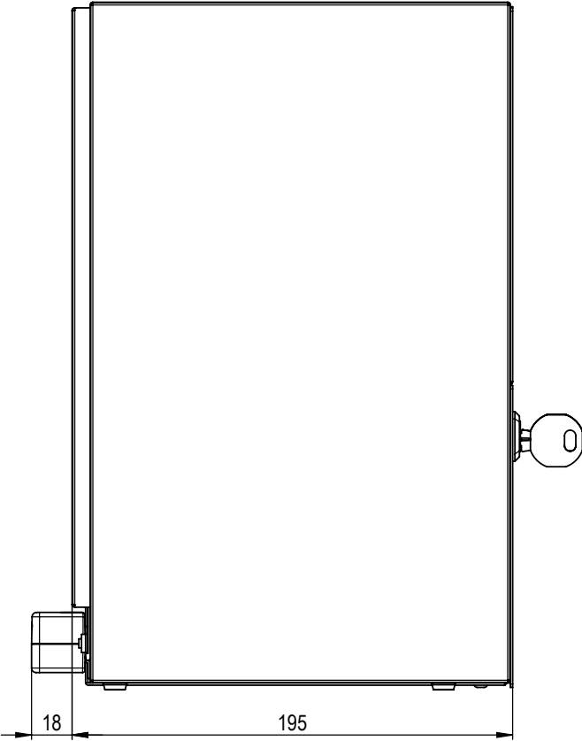
Zijaanzicht
